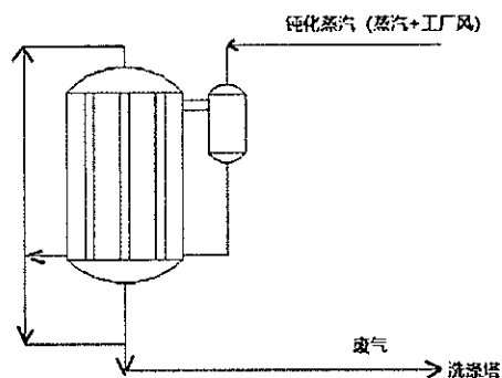
钝化流程示意图
