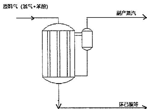
正常工艺流程
